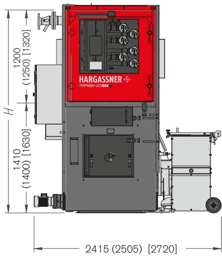
Maßangaben in mm für Magno-VR 250 (Maßangaben in mm für Magno-VR 300–395) [Maßangaben in mm für Magno-VR 399–600]
