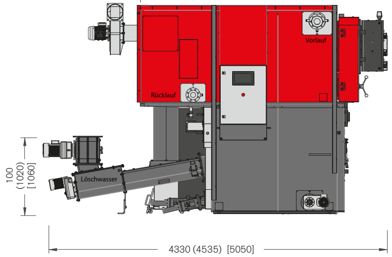
Maßangaben in mm für Magno-VR 250 (Maßangaben in mm für Magno-VR 300–395) [Maßangaben in mm für Magno-VR 399–600]
