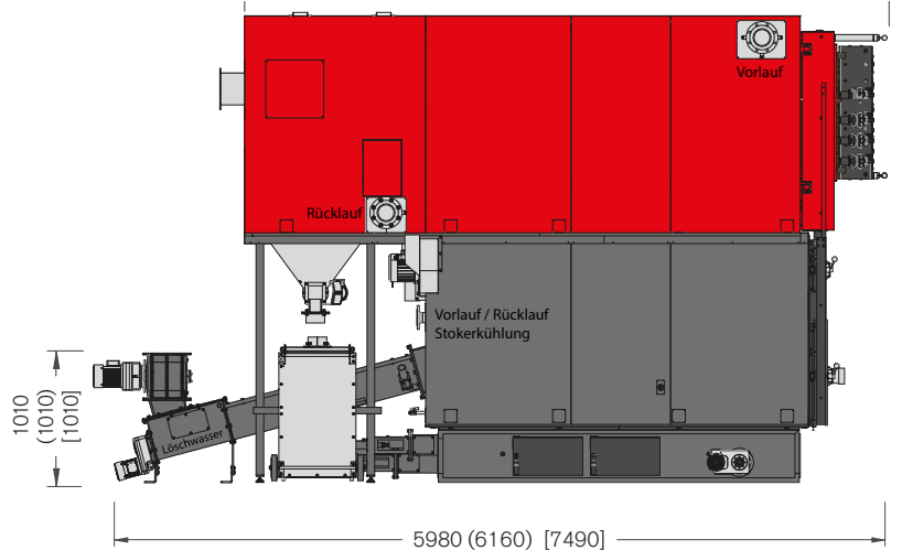
Maßangaben in mm für Magno-SR 800–1.200 (Maßangaben in mm für Magno-SR 999–1.400) [Maßangaben in mm für Magno-SR 2.000–2.500]
