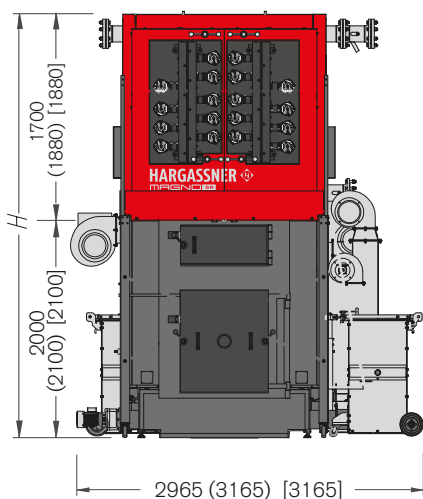
Maßangaben in mm für Magno-SR 800–1.200 (Maßangaben in mm für Magno-SR 999–1.400) [Maßangaben in mm für Magno-SR 2.000–2.500]
