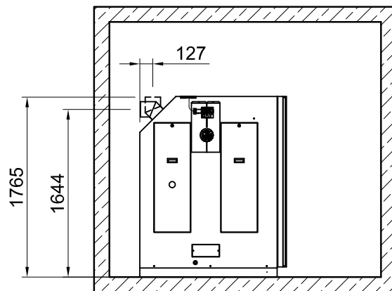
Coude de tuyau de fumée à 45° (par client)
