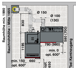
Neo-HV mit Nano-PK rechts, RR waagr.
