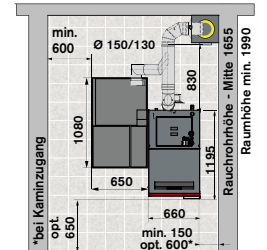
Neo-HV mit Smart-PK links, RR waagr.
