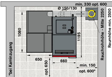
Neo-HV mit Smart-PK links, RR senk.
