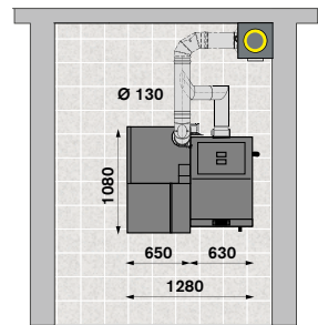
Smart-HV mit Smart-PK links, RR waagr.
