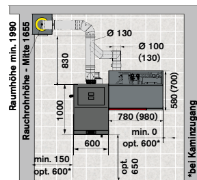
Smart-HV mit Nano-PK rechts, RR waagr.
