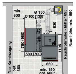
Neo-HV mit Nano-PK links, RR waagr.
