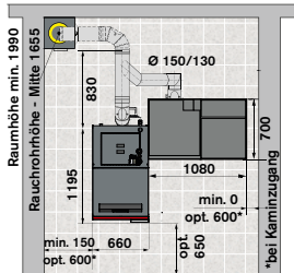
Neo-HV mit Smart-PK rechts, RR waagr.
