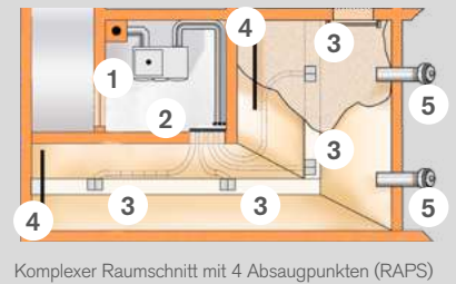
Komplexer Raumschnitt mit 4 Absaugpunkten (RAPS)
