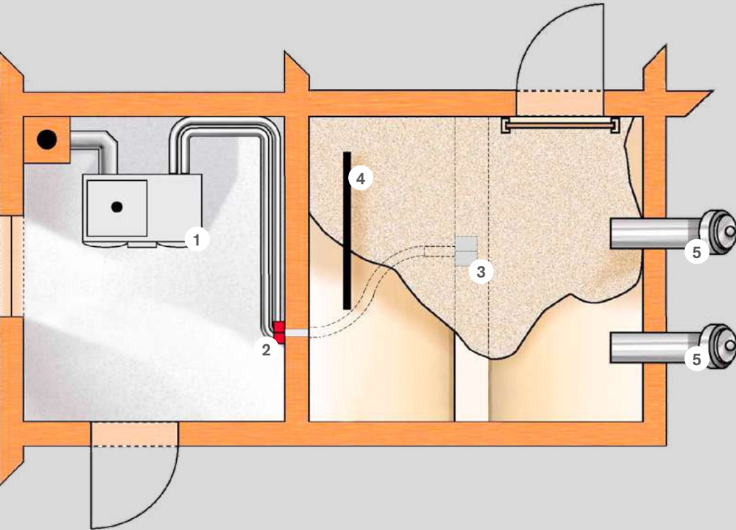
Komplexer Raumschnitt mit 4 Absaugpunkten (RAPS)
