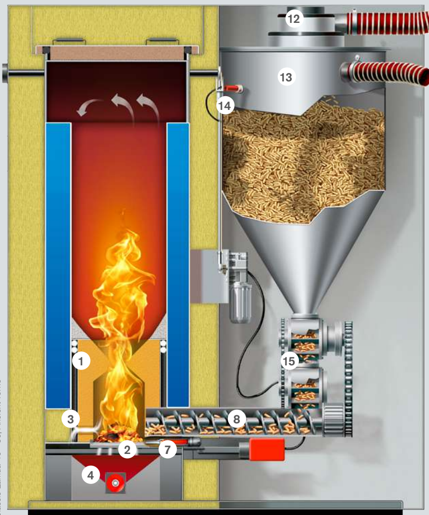
Classic Lamda 40–60, Ansicht vorne
