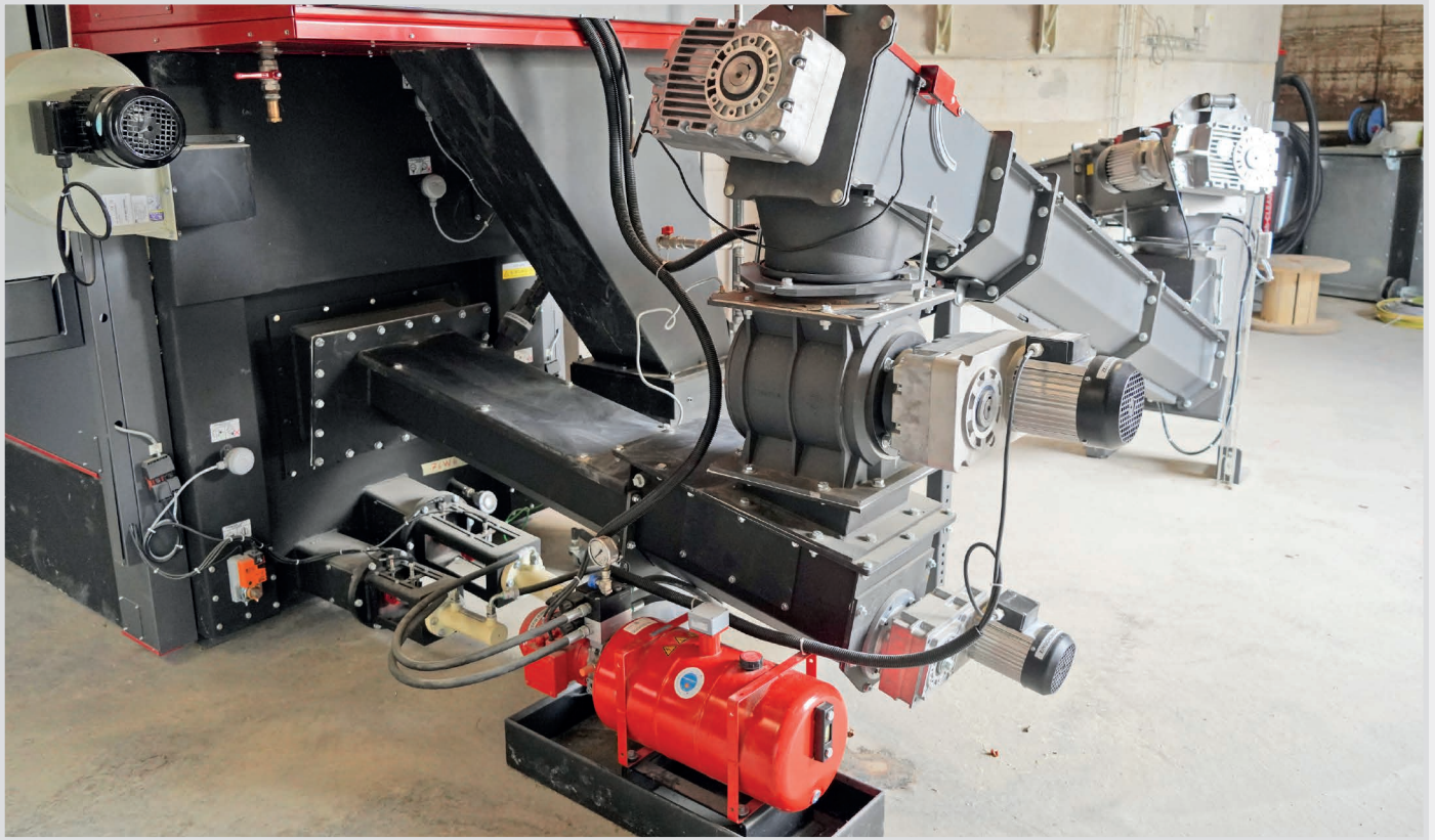
Die Zelleradschleuse für eine 100%ige Rückbrandsicherheit mit der Einschubschnecke. Und das Hydraulikaggregat für den Vorschubrost und die Unterrostentaschung.
